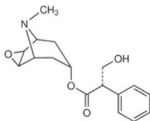
Hyoscina
