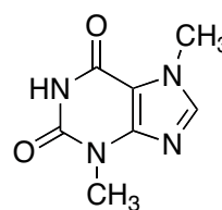
Teobromina
