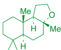
Ambrox
