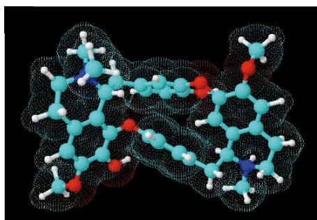
Tubocurarina
