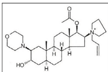
Rocuronio
