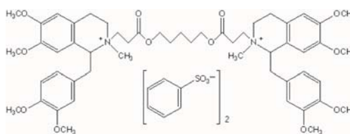
Atracurio
