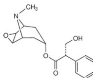
Hyoscina (escopolamina)
