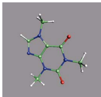
Cafeína
