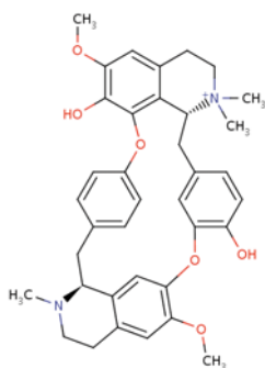
Tubocurarina
