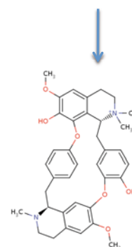
King (1935, estructura)
