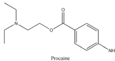
Novocaína (Sintética)
