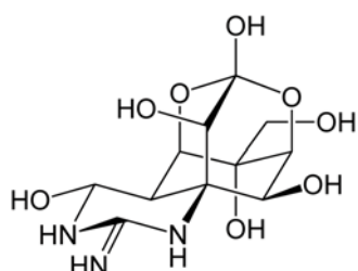
Tetrodotoxina (neurotoxina)
