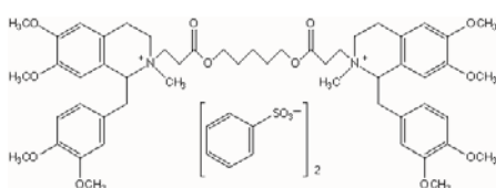
Bloqueantes sintéticos
