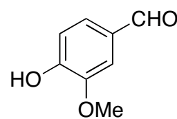
Vainillina
